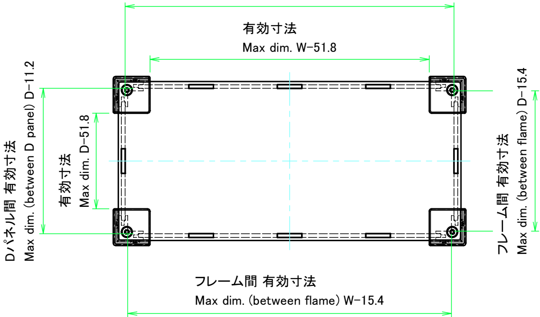
Wパネル間 有効寸法 Max dim. (between W panel) W-11.2
